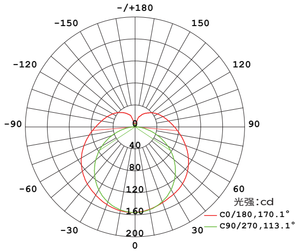
配光曲线
